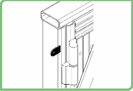
3.3 Orejetas modo tapajuntas
