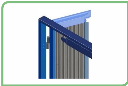
Detalle superior
