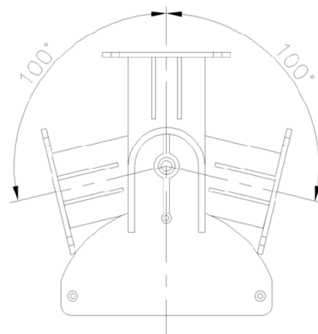
POSICIONES DE MONTAJE (VISTA EN PLANTA)
